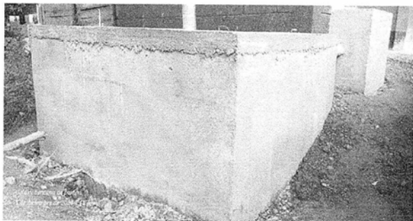
Foto 3: fosa septica terminada
